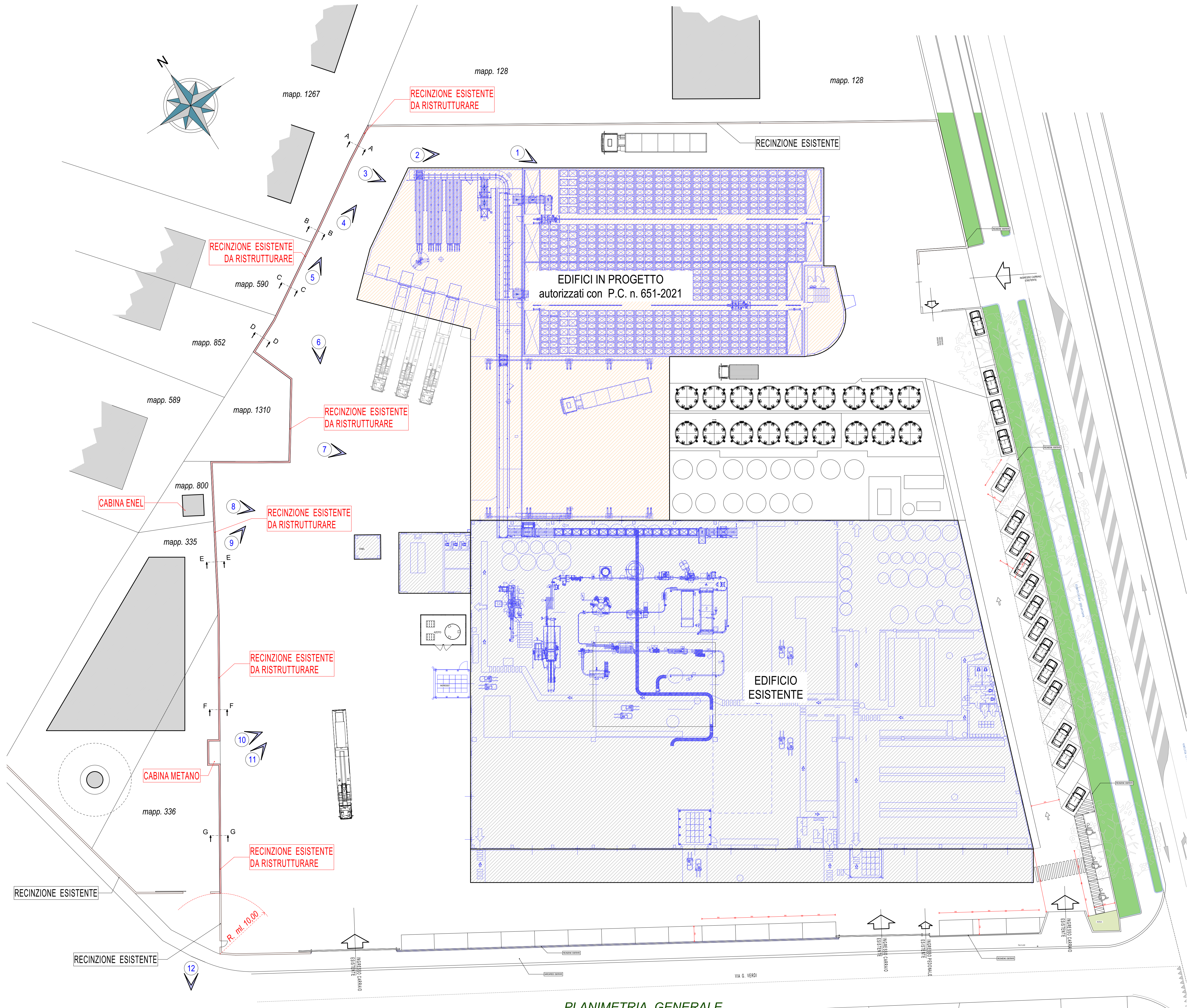
PLANIMETRIA GENERALE scala 1/300
